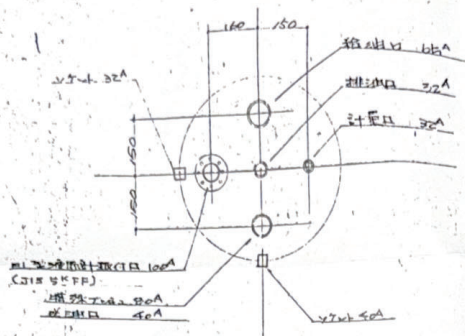
マンホール蓋詳細図 1:10
