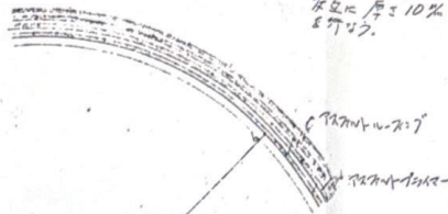
タンク外面保護仕様図
